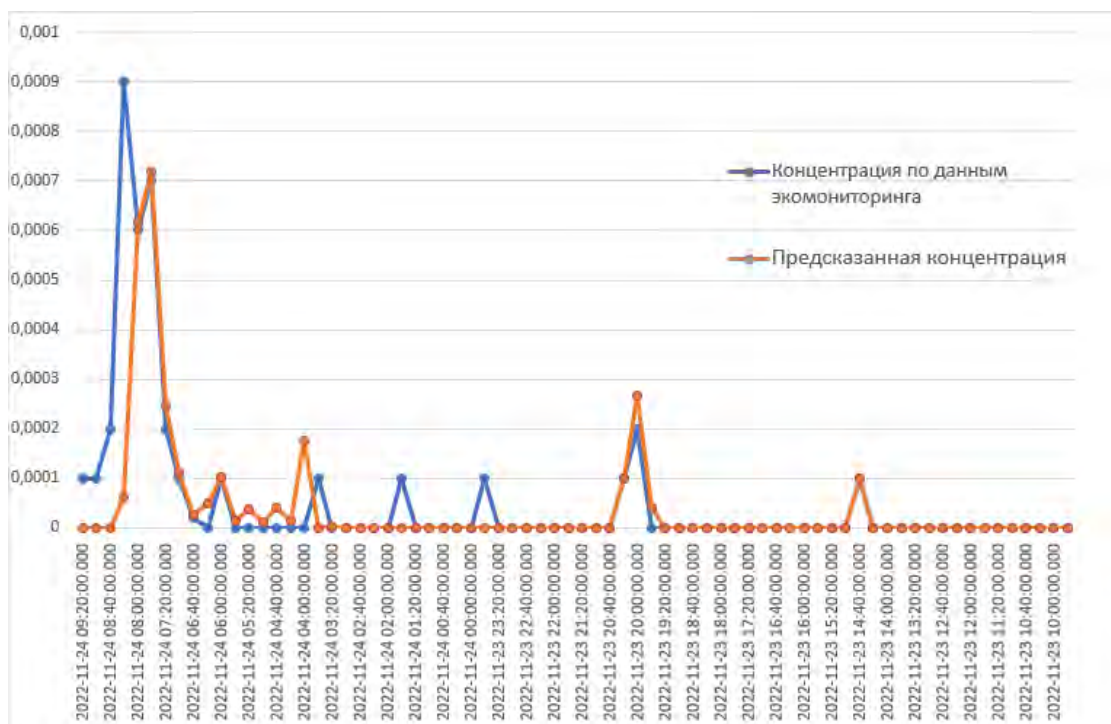
Рис. 3. Сравнительная диаграмма измеренных и полученных путем моделирования значений концентрации
