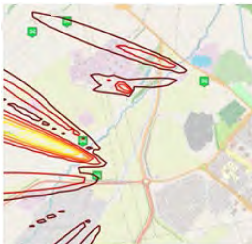
Рис. 2. Распространение сероводорода 23-24 ноября 2022, класс стабильности атмосферы E
