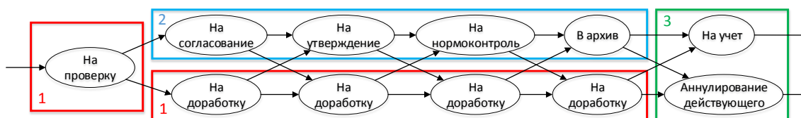
Рисунок 7 – ИНС-модель традиционного маршрута согласования ТД с выделенными группами элементов для улучшения
