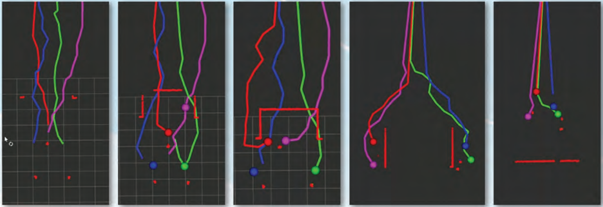
Рис. 16. Моделирование прохождения группой препятствия П-образного типа Fig. 16. Simulation of UUV group overcoming a П-shaped obstacle
