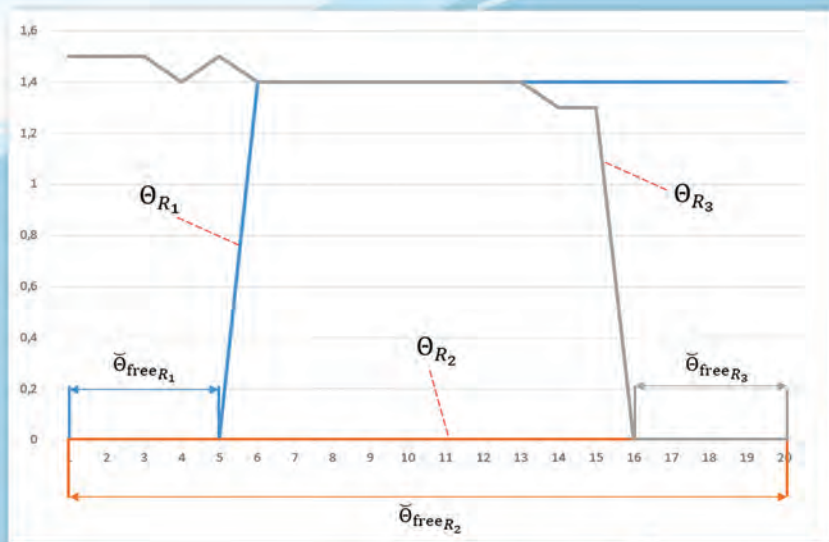
Рис. 7. Пример оценки общего поля видимости группы \Theta_g (для второй ситуации из рис. 5)
