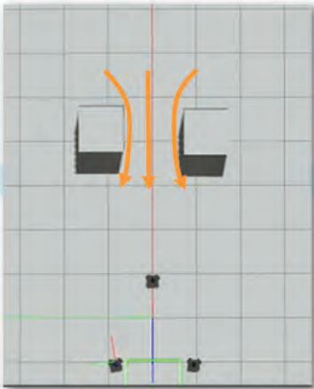
Рис. 17. Пример сцены моделирования с областью течения, противонаправленного движению Fig. 17. Example of simulation – cross-current conditions
