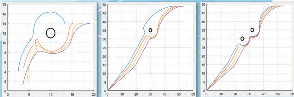
Рис. 3. Пример обхода статических препятствий группой агентов за счет применения системы визуального потенциального поля
