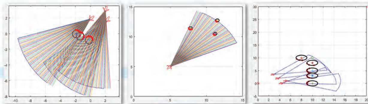
Рис. 2. Пример работы модуля системы технического зрения (одного агента) и обнаружения облака точек (красные точки) группой морских робототехнических комплексов
