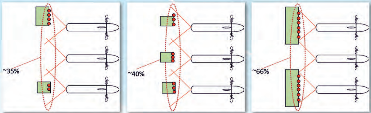
Рис. 4. Составление общего поля видимости и принятия решения о реконфигурации группой автономных необитаемых подводных аппаратов
