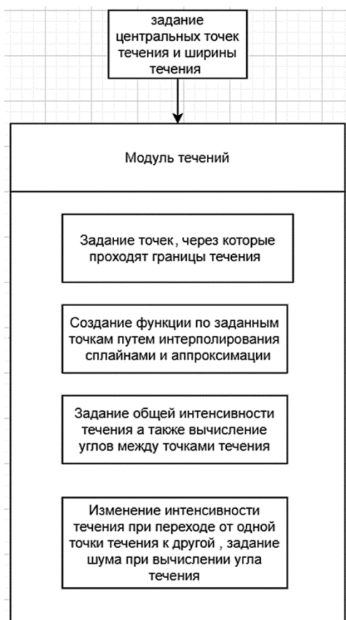
Рис. 9. Блок-схема процесса построения структуры течения Fig. 9. Flow chart of current structure development algorithm
