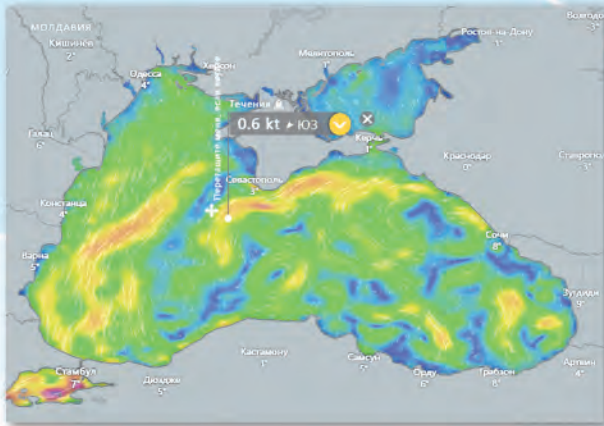
Рис. 8. Карты течений Черного моря Fig. 8. Maps of Black Sea currents
