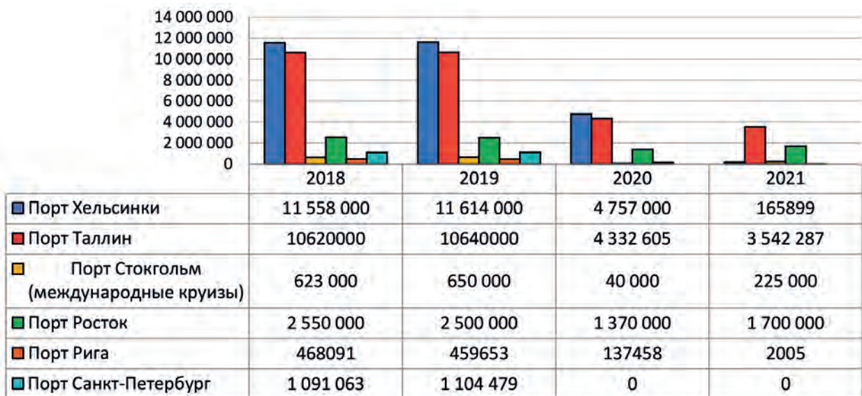
Рис. 2. Анализ пассажиропотока морских пассажирских портов Балтийского моря в период 2018–2022 гг.
