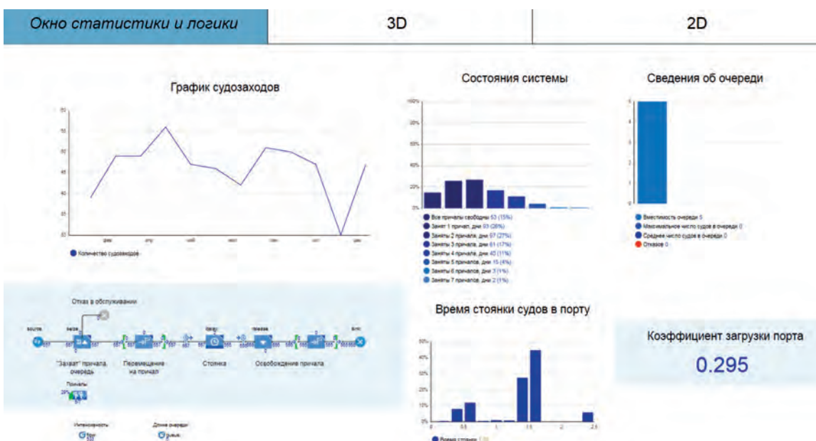
Рис. 5. Практическая реализация в AnyLogic графиков функции интенсивности паромных и круизных судов
