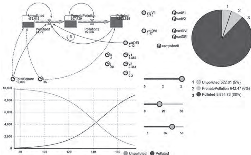
Рис. 4. Панель настроек модели и визуализации результатов прогона Fig. 4. Board of model setting and run outcome visualization
