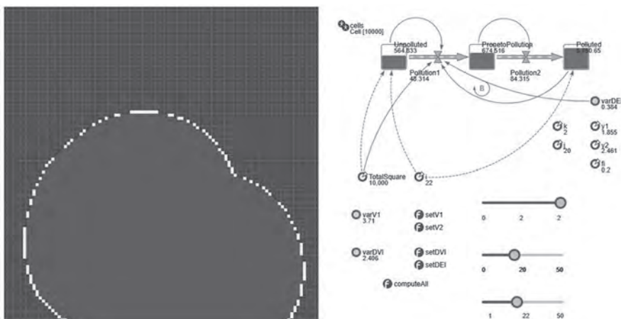
Рис. 5. Визуализация прогона модели в Муровом пространстве Fig. 5. Visualization of model run in Murovian space
