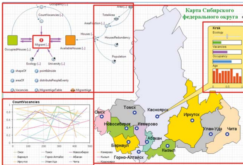
Рис. 4. Общий вид имитационной модели в среде AnyLogic
