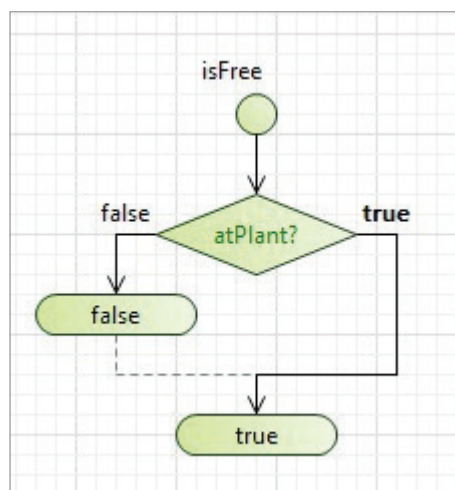
Рис. 2.57. Функция isFree
