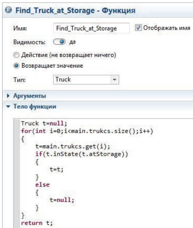
Рис. 6.11. Функция Find_Truck_at_Storage
