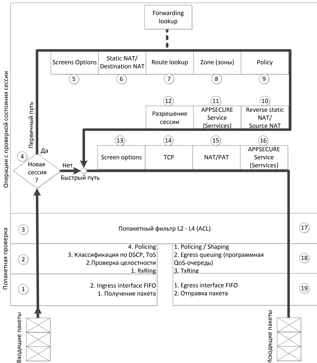
Рисунок А.2 – Схема задержки при обработке пакетов Juniper SRX предыдущего поколения
