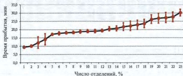
Рисунок 17 – Распределение времени прибытия к исследуемому объекту при возникновении ситуации одновременного обслуживания двух крупных ЧС (по результатам моделирования)
