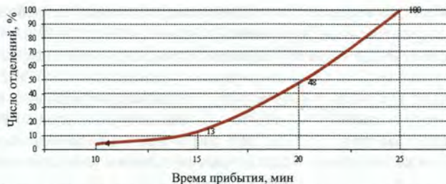
Рисунок 18 – Кумулята времени прибытия к исследуемому объекту при возникновении ситуации одновременного обслуживания двух крупных ЧС (по результатам моделирования)
