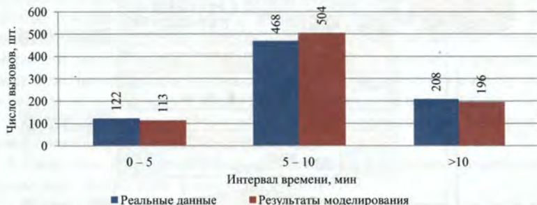
Рисунок 9 – Распределение реальных данных с результатами моделирования времени прибытия к месту вызова
