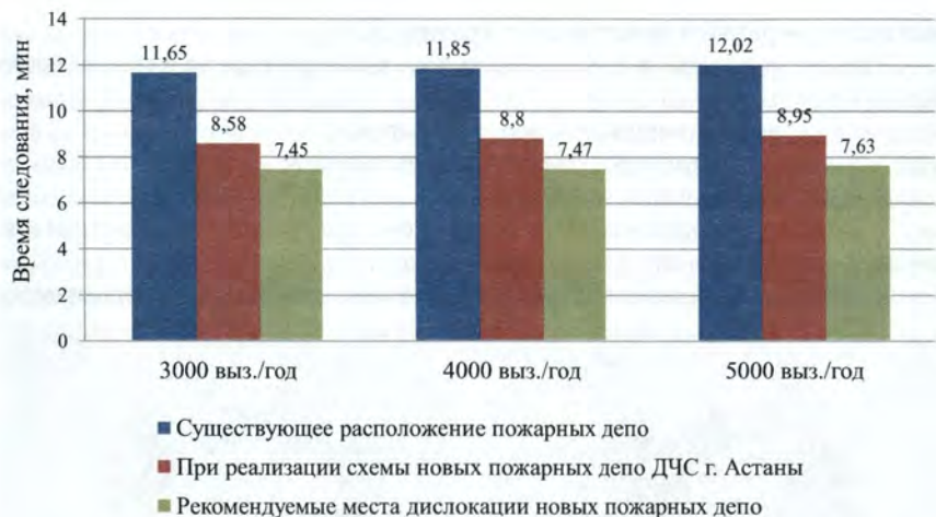
Рисунок 23 – Распределение времени следования ПСГ к местам вызовов (по результатам моделирования)
