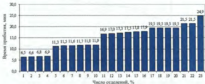
Рисунок 13 – Распределение времени прибытия для различного числа оперативных отделений к исследуемому объекту при текущих параметрах оперативной обстановки (по результатам моделирования)
