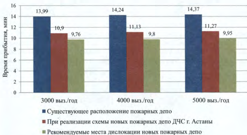
Рисунок 24 – Распределение времени прибытия ПСГ к местам вызовов (по результатам моделирования)
