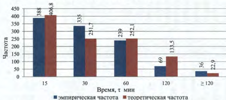
Рисунок 4 – Гистограмма эмпирического и теоретического распределений длительности времени обслуживания вызовов ПСП в городе
