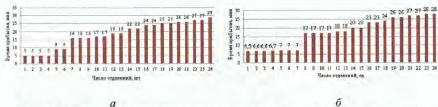
Рисунок 6 – Распределение реального времени прибытия различного числа оперативных подразделений при крупных пожарах:
