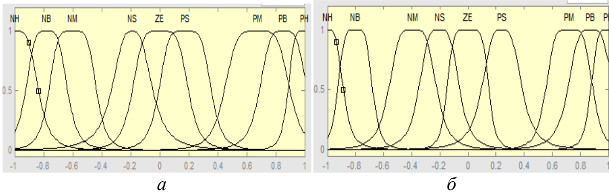
Рисунок 5 – ФП переменных Pr_{t_n} (a) и Pr_{t_{n-1}} (б) после адаптации
