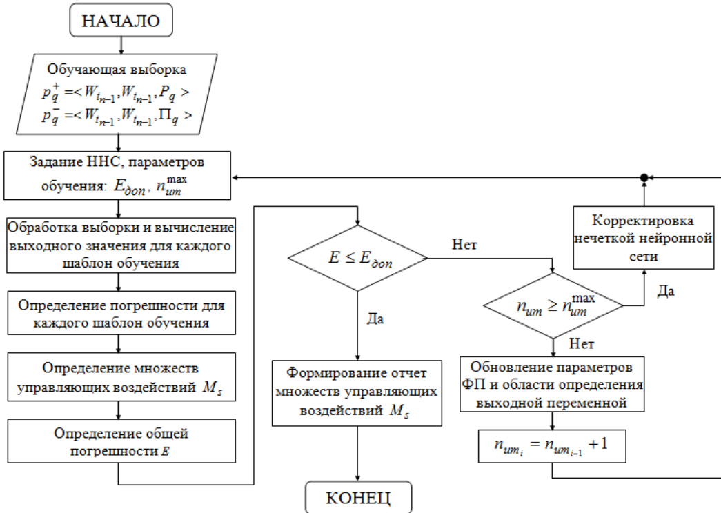
Рисунок 4 – Метод адаптации нечёткой системы управления трафиком информационно-коммуникационных пакетов, основанной на использовании ННС
