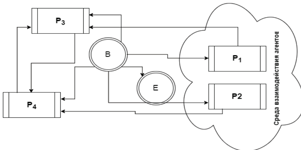
Графовая модель переходов для агента пассажиров: V – точка старта агента; E – завершение функционирования агента; P 1 , P 2 , P 3 , P 4 – континуум процедур процессов агента; U – переходы между отдельными состояниями агента
