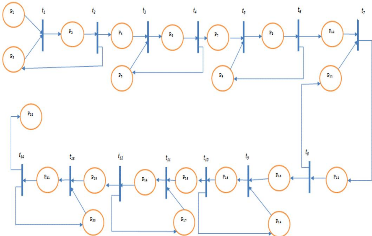
Рис. 5. Сеть Петри, моделирующая технологический процесс производства твердых лекарственных форм (разработано авторами)
