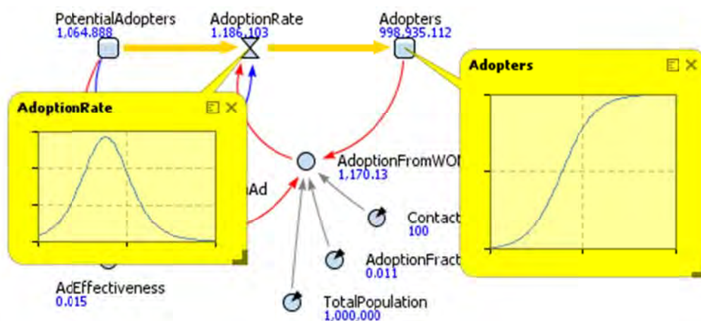
Рис. 3.16. Модель AnyLogic, использующая метод системной динамики
