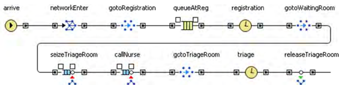
Рис. 3.14. Сетевое моделирование в AnyLogic
