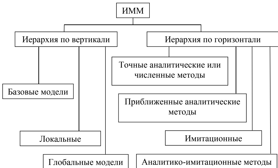
Рис. 1.3. Иерархическое многоуровневое моделирование
