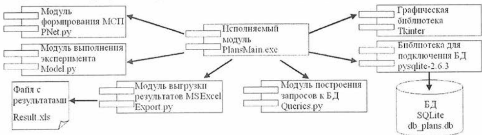
Рисунок 6 – Модульная структура программного средства формирования производственных расписаний
