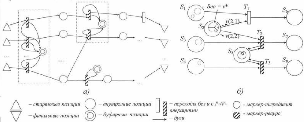
Рисунок 1: а) Пример графического отображения фрагмента модифицированной сети Петри; б) Пример определения разрешимости срабатывания вершин-переходов по весу маркеро-ингредиентов
