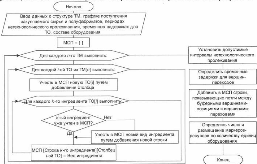
Рисунок 4 – Общая схема алгоритма построения модифицированной сети Петри при формировании производственных расписаний
