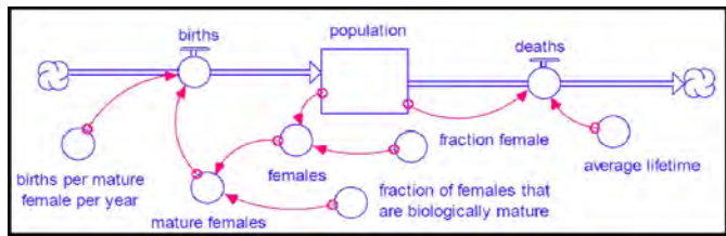
б) системно-динамическая модель роста популяции, построенная в системе Stella [23]
