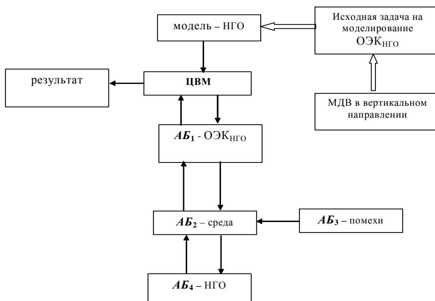
Рис. 2. Имитационная модель измерения высоты нижней границы облаков
