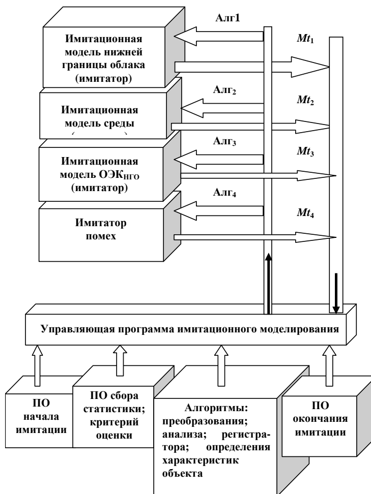
Рис. 3. Блок-схема имитационного моделирования оптико-электронного комплекса измерения высоты нижней границы облака способом просмотра активностей
