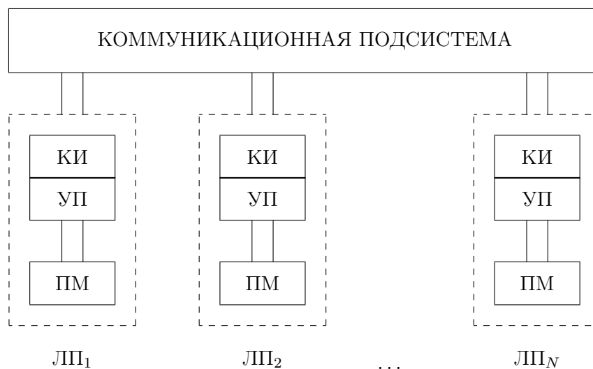
Рис. 2. Схема выполнения распределенной модели: ЛП — логический процесс, ПМ — подмодель, УП — управляющая программа, КИ — коммуникационный интерфейс.
